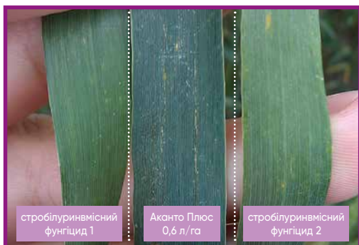
Фото 2. Виразений «зелений ефект» Аканто Плюс® 0,6 л/га у порівнянні з іншими стробілуриновмісними фунгіцидами у фазу прапорцевого листка озимої пшениці через 16 днів після обробки, Харківська обл., 2018
